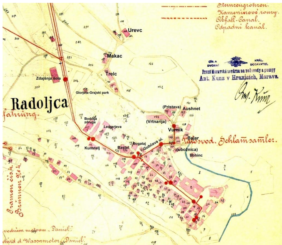
Načrt vodovoda, 1902 Vir: 100 let Komunale v Radovljici
