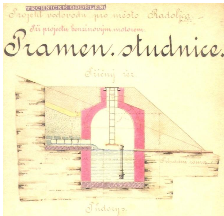
Detail iz »Projekta vodovoda za mesto Radovljica«, 1902 Vir: 100 let vodovoda v Radovljici (izdala: Komunala Radovljica)
