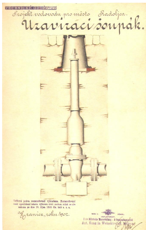
Detail iz »Načrta vodovoda za mesto Radovljica«, 1902 Vir: 100 let vodovoda v Radovljici (izdala: Komunala Radovljica)
