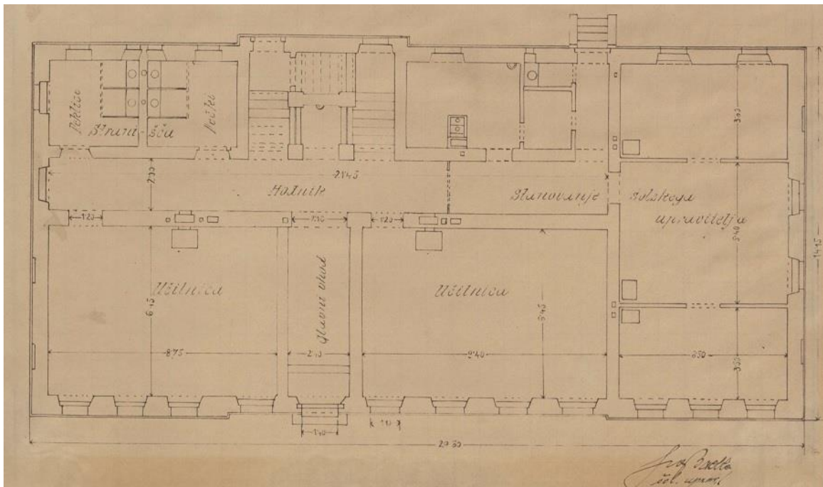
Načrt šole – pritličje, 1904 Vir: sistory.si / Slovenski šolski muzej Ljubljana
