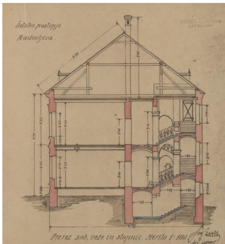
Šola – prerez sob, veže in stopnic, 1904 Vir: sistory.si / Slovenski šolski muzej Ljubljana
