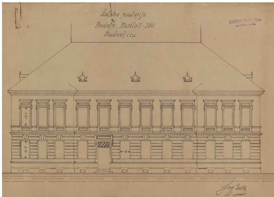
Pročelje šolske stavbe, 1904
